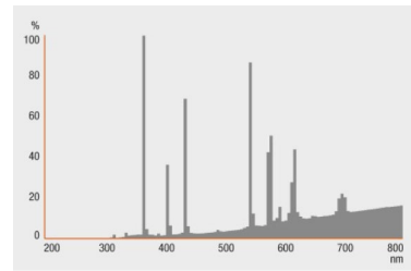
HWL 250 W 235 V E40, HWL 500 W 235 V E40
