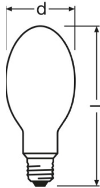
HWL 160 W 220 V E27, HWL 250 W 235 V E40, HWL 500 W 235 V E40
